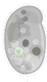
Colpidium (bobovka)
