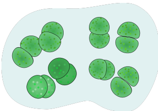
Limnococcus
