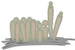
Chamaesiphon
