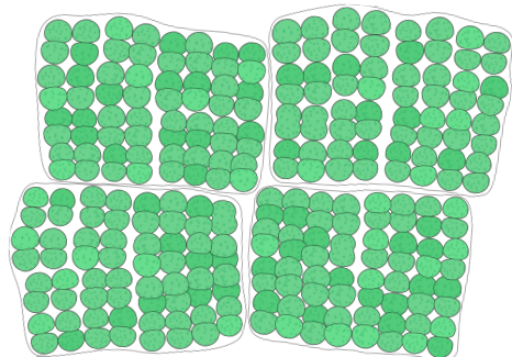
Merismopedia
