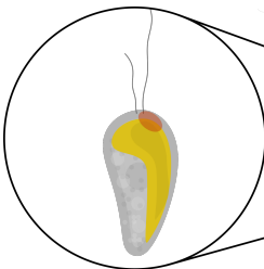
Uroglena
