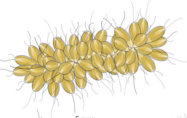
Synura
