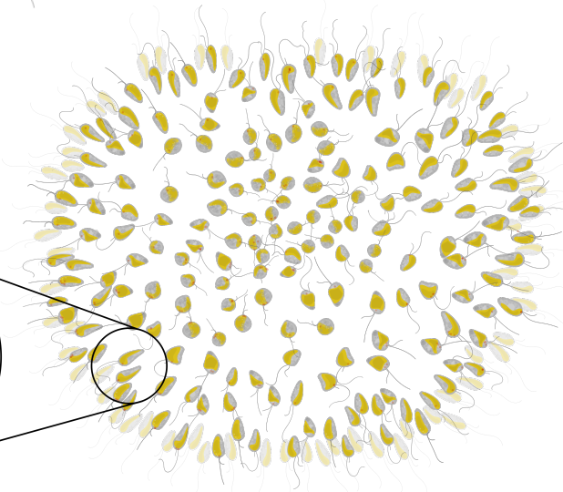
Uroglena
