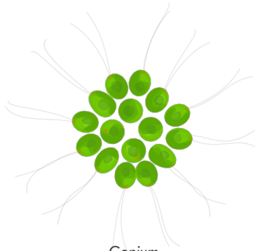
Gonium
