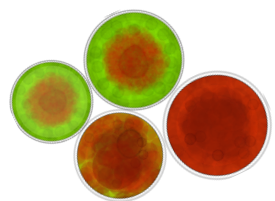
Haematococcus
