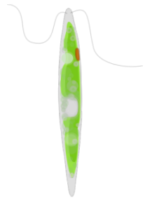
Chlorogonium
