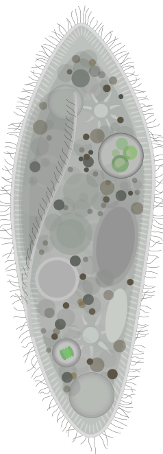
Paramecium caudatum
