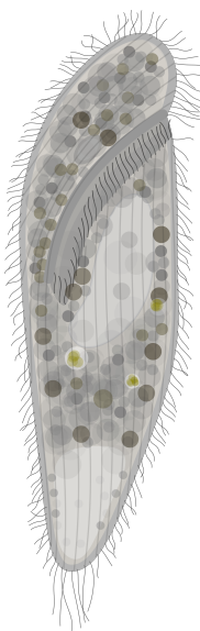
Metopus
