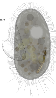
Pleuronema
