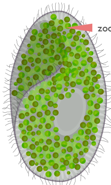
Paramecium bursaria
