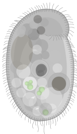
Colpidium
