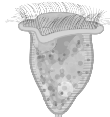
Vorticella
