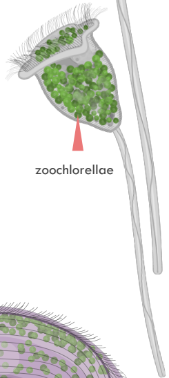
Vorticella
